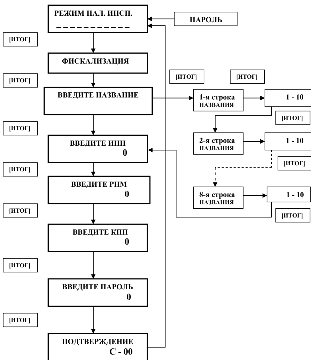
Рис.2. Структурная схема фискализации ККМ.
